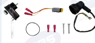
Kostal - M27 - 2 Pin + Deutsch
